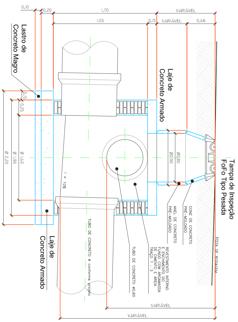
POÇO DE VISITA ESC.: 1/30
